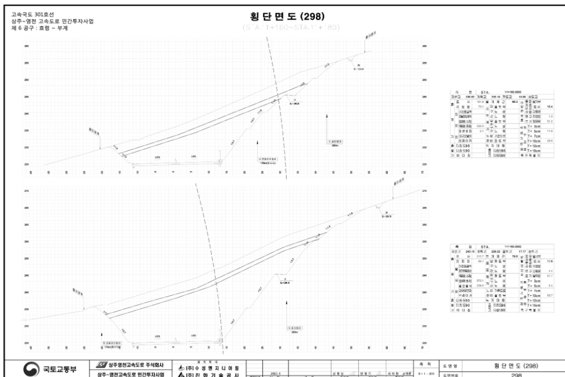
【그림 39.4】 표준횡단면도
