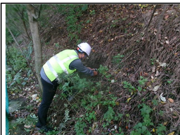
절리면 경사/경사방향 측정
