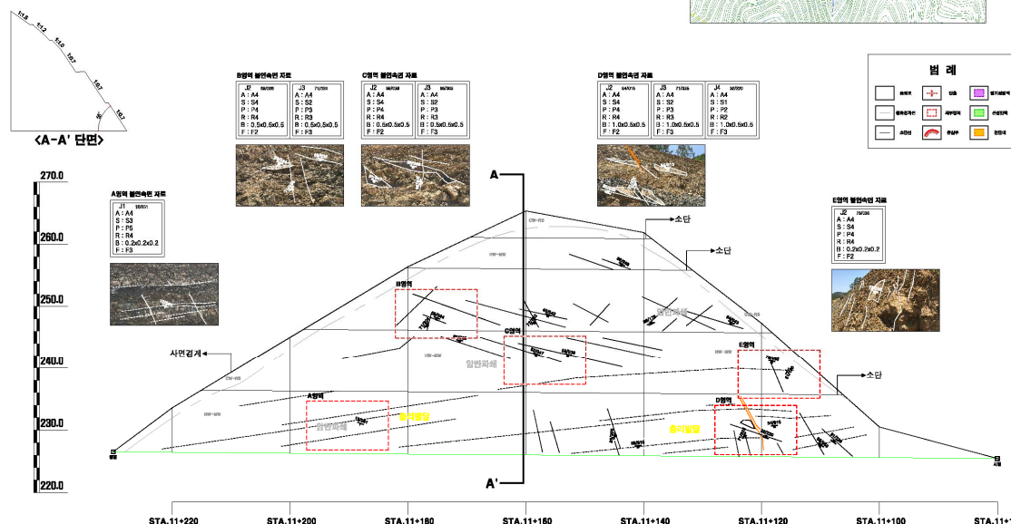
【그림 39.14】 영천절토39 검토대상 비탈면구간
